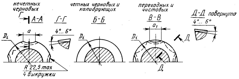
Форма зубьев и расположение выкружек на зубьях:
